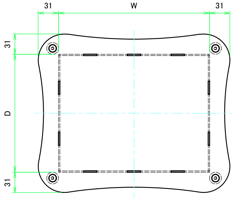
上カバー / Top cover
